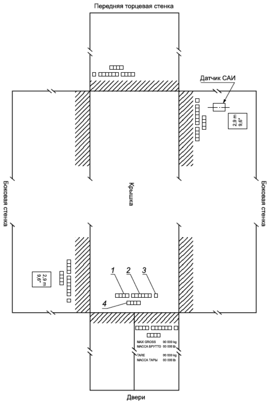
1 - код владельца; 2 - серийный номер; 3 - контрольное число; 4 - код размера и типа Рисунок Б.1 - Схема нанесения маркировки на внешнюю поверхность мобильного (инвентарного) здания
